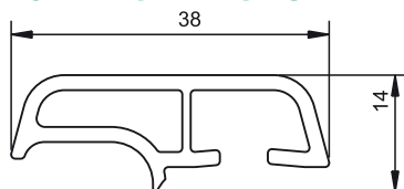
Bagheta acoperire TP5206 Copribattuta TP5206 Lefedettség párkányfogadó TP-5206
