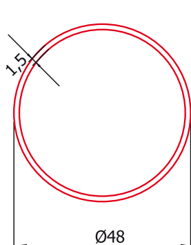
Armătură R508/15 Greutate: 1,72 kg/m Rinforzo R508/15 Peso 1,72 kg/m Merevítés R508/15 Súly 1,72 kg/m
