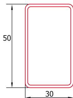
Armătură R3050/20 Greutate: 2,346 kg/m Rinforzo R3050/20 Peso 2,346 kg/m Merevítés R3050/20 Súly 2,346 kg/m
