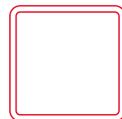
Armătură R2828/15 Greutate: 1,212 kg/m Rinforzo R2828/15 Peso: 1,212 kg/m Merevítés R2828/15 Súly 1,212 kg/m
