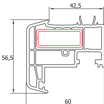
Bordură ușă TP-4703 Scambio battuta porta TP-4703 Ajtó váltószárny TP-4703
