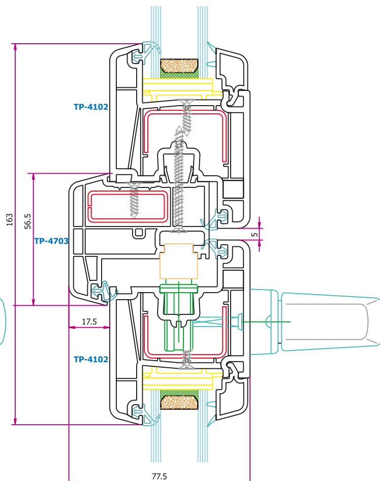
Secțiune mediană cu bordură ușă Sezione mediana a scambio battuta porta Keresztmetszet váltószárnyal
