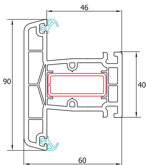
Montant TP4103 - standard Montant TP4103 - Eco Montante TP4103 - standard Montante TP4103 - Eco Osztó TP4103 - standard Osztó TP4103 - Eco
