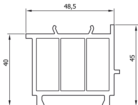
Cuplaj perete 45 mm TP5301 Accoppiatore per davanzale 45mm TP5301 Toktoldó 45mm TP5301
