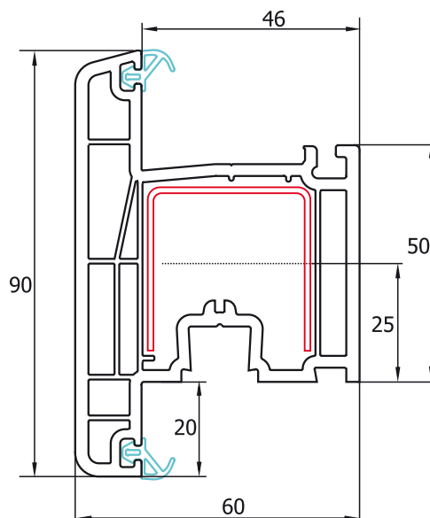
Cercevea intermediara pentru uși TP4106 - standard Anta intermedio per porta TP4106 - standard Ajtó Üvegezőléc közbűlső TP-4706
