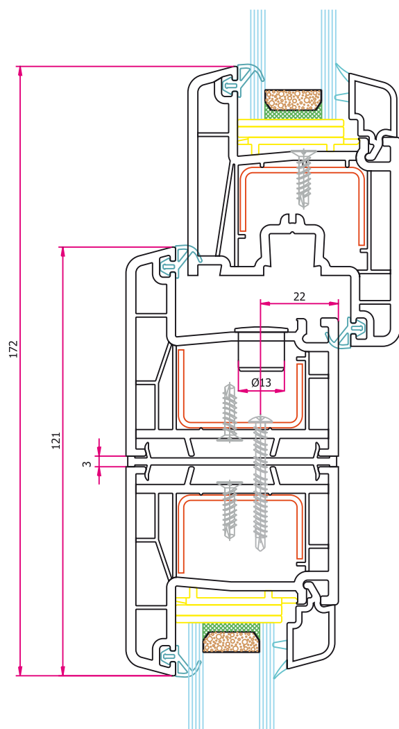
Cuplare simplă Accoppiamento semplice Egyszerű sorolás
