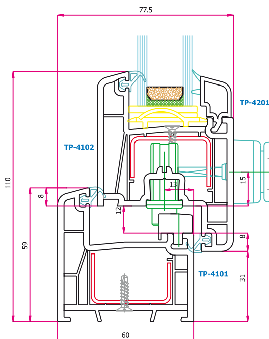
Secțiune latura inferioară confecție fixă Sezione lato inferiore confezione fisso Alsó oldal keresztmetszete - fix szerkezet
