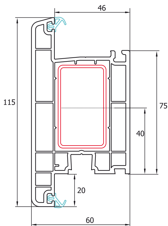
Cercevea ușă TP4702 - standard Cercevea ușă TP4702 - Eco Anta porta TP4702 - standard Anta porta TP4702 - Eco Ajtó Üvegezőléc TP-4702 - standard Ajtó Üvegezőléc TP-4702 - Eco
