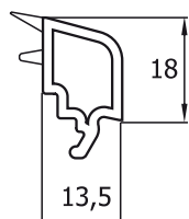
Bagheta 24 mm TP-4201 Fermavetro doppio labro 24 mm TP-4201 Üvegezőléc 24 mm TP4201
