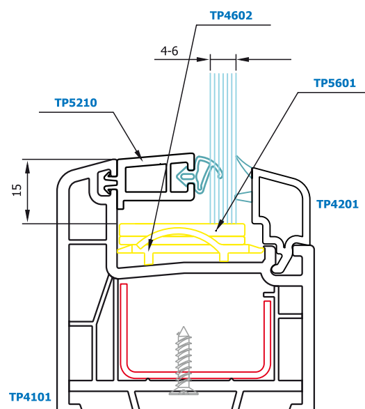
Secțiune cu geam simplu și baghetă completare Semplice vetro sezione e completamento bacchetta Keresztmetszet a Befejezése párkányfogadó
