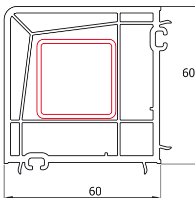
Cuplaj 90° TP4304 Accoppiamento 90° TP4304 Csatlakozó 90° TP-4304
