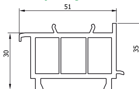
Cuplaj perete 35 mm TP5310 Accoppiato a davanzale 35 mm TP5310 Toktoldó 35mm TP5310
