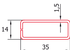
Armătura R505/15 Greutate: 1,035 kg/m Rinforzo R505/15 Peso: 1,035 kg/m Merevítés R505/15 Súly 1,035 kg/m
