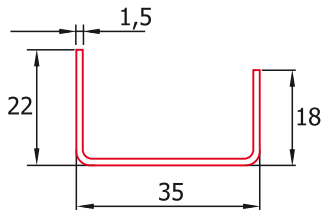
Armătură R3522/15 Greutate: 0,814 kg/m Rinforzo R3522/15 Peso 0,814 kg/m Merevítés R3522/15 Súly 0,814 kg/m
