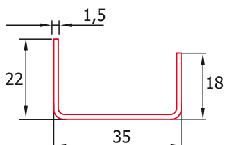
Armătura R3522/15 Greutate: 0,814 kg/m Rinforzo R3522/15 Peso: 0,814 kg/m Merevítés R3522/15 Súly 0,814 kg/m
