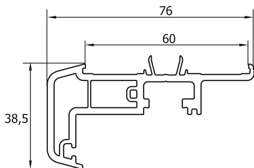
Bordură fereastră TP-4104 Scambio battuta finestra TP-4104 Ablak váltószárny TP-4104
