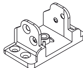
Conector montant 30127 Connettore montante 30127 Osztóbekötő 30127
