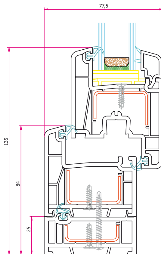
Cuplare cu profil de adăugare 25mm Accoppiamento con profilo aggiunta 25mm Toksorolás toktoldóval 25mm
