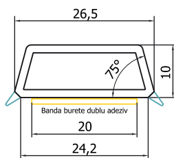
Bagheta Ornament P TP4202 Bacchetta Ornamento P TP4202 Ornament üvegezőléc P TP4202
