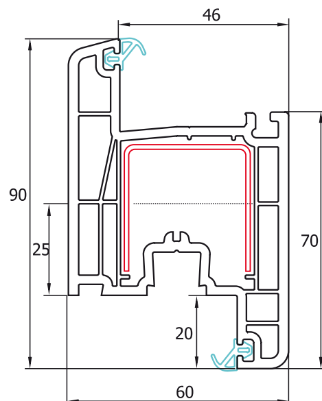
Cercevea intermediară pentru uși TP4105 - standard Anta intermedio per porta TP4105 - standard Ajtó Üvegezőléc közbűlső TP-4705
