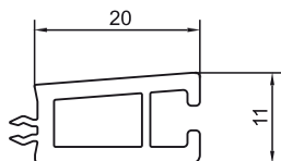
Bagheta completare TP5210 Fermavetro per vetro singolo TP5210 Befejezése párkányfogadó TP-5210
