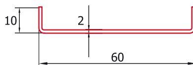
Armătură R6010/20 Greutate: 1,17 kg/m Rinforzo R6010/20 Peso: 1,17 kg/m Merevítés R6010/20 Súly 1,17 kg/m
