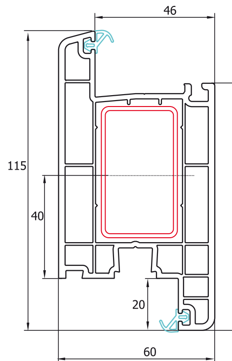
Cercevea ușă TP4701 - standard Cercevea ușă TP4701 - Eco Anta porta TP4701 - standard Anta porta TP4701 - Eco Ajtó Üvegezőléc TP-4702 - standard Ajtó Üvegezőléc TP-4702 - Eco
