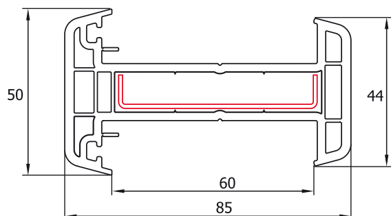
Profil de dilatare TP4307 Profilo espansione TP4307 Dilatációs profil TP-6307
